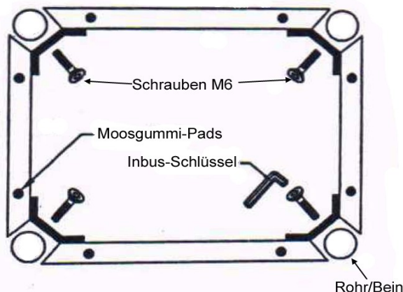
Drauf-Sicht
